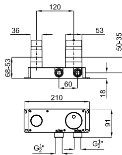
Internal part for wall basin mixer with Ø35 mm ceramic cartridge. 1/2" connectors. Corps interne pour mitigeur encastré lavabo avec cartouche céramique de Ø35 mm. Connexions de 1/2".
