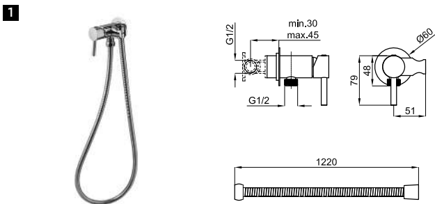
1 External parts of mixer for sanitary showers. Wall bracket with outlet elbow and hose included. Parties extérieures robinet Mélangeur pour douchette sanitaire. Inclus support mural avec prise d'eau et flexible.
