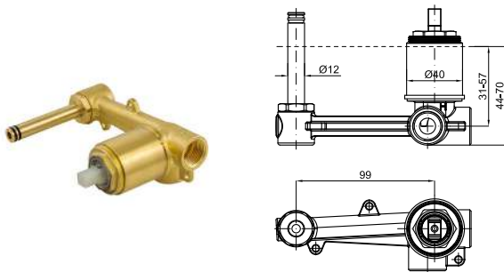
Internal part for wall basin mixer with Ø35 mm ceramic cartridge. 1/2" connectors. Corps interne pour mitigeur encastré lavabo avec cartouche céramique de Ø35 mm. Connexions de 1/2".
