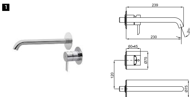
1 Single lever basin mixer trim kit. Without pop up waste. Flow rate 5 L/min at 3 bar. Partie externe mitigeur encastré lavabo. Sans bonde. Le débit à 3 bars est de 5 L/min.
